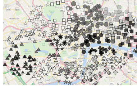
Figure 3 – Clusters de stations source dessinées sur la carte de Londres. Il y a un symbole gris par cluster.
